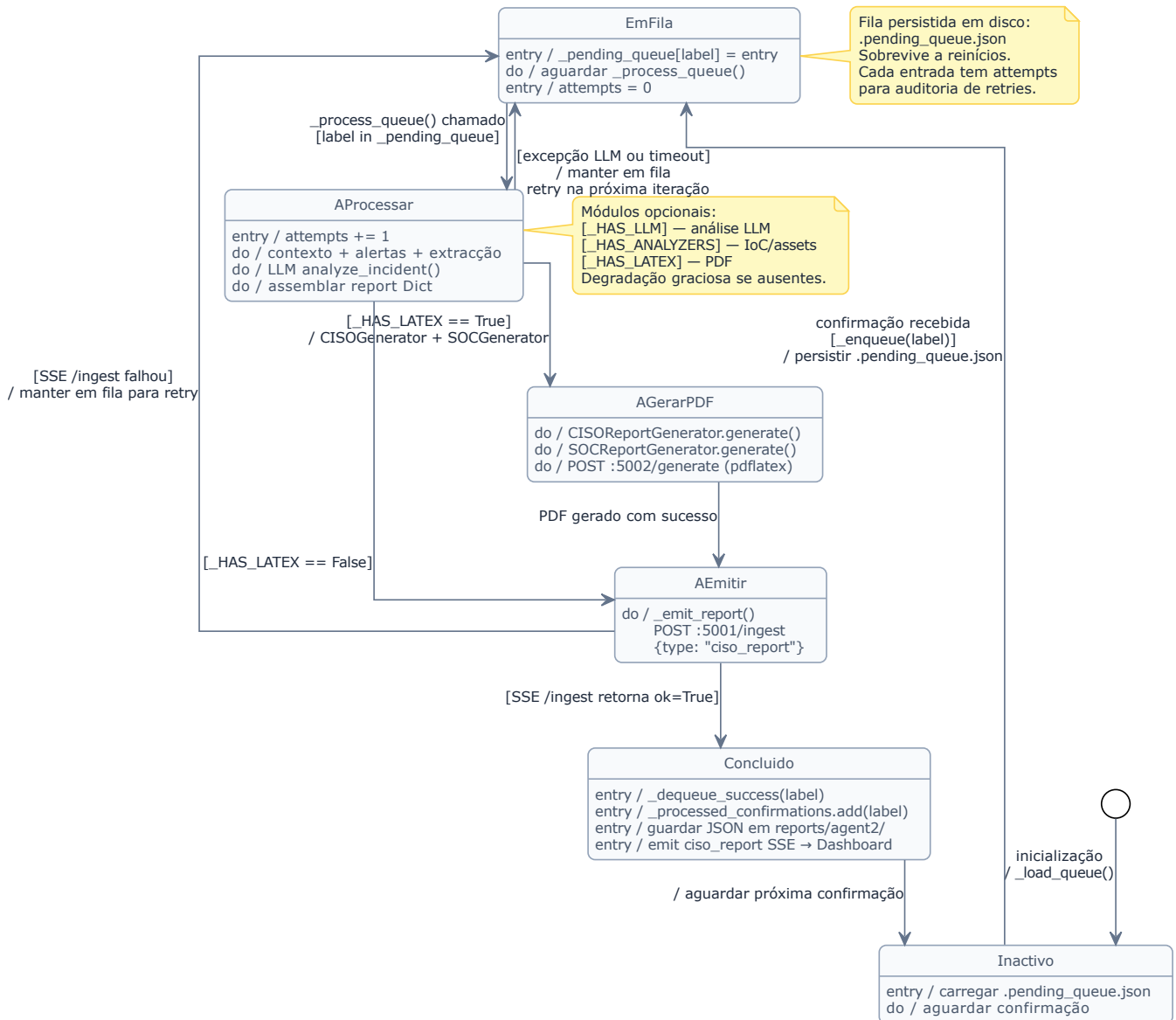
Figure 1: Máquina de Estados: Ciclo de Vida do Relatório
